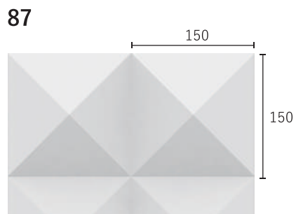
Bタイプ・B+Bタイプ 断面図
