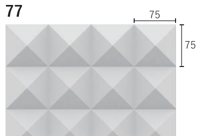
Bタイプ・B+Bタイプ 断面図
